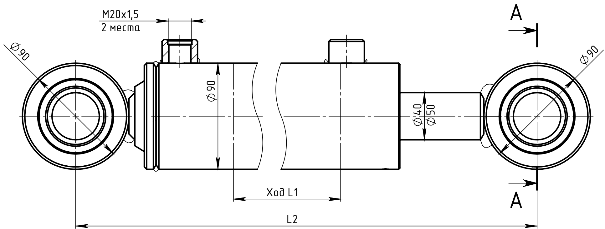
Исполнение 2
