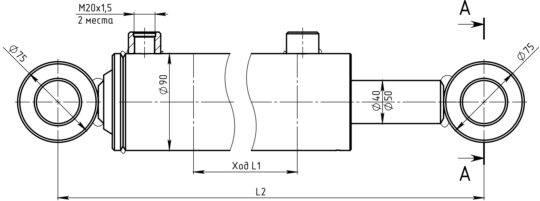
Исполнение 1
