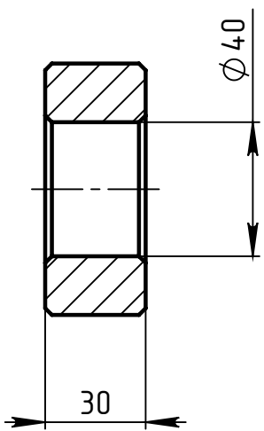
A-A
