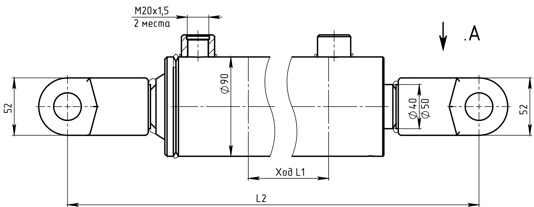
Исполнение 3
