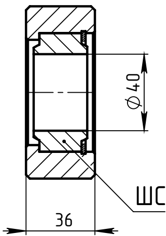
A-A
