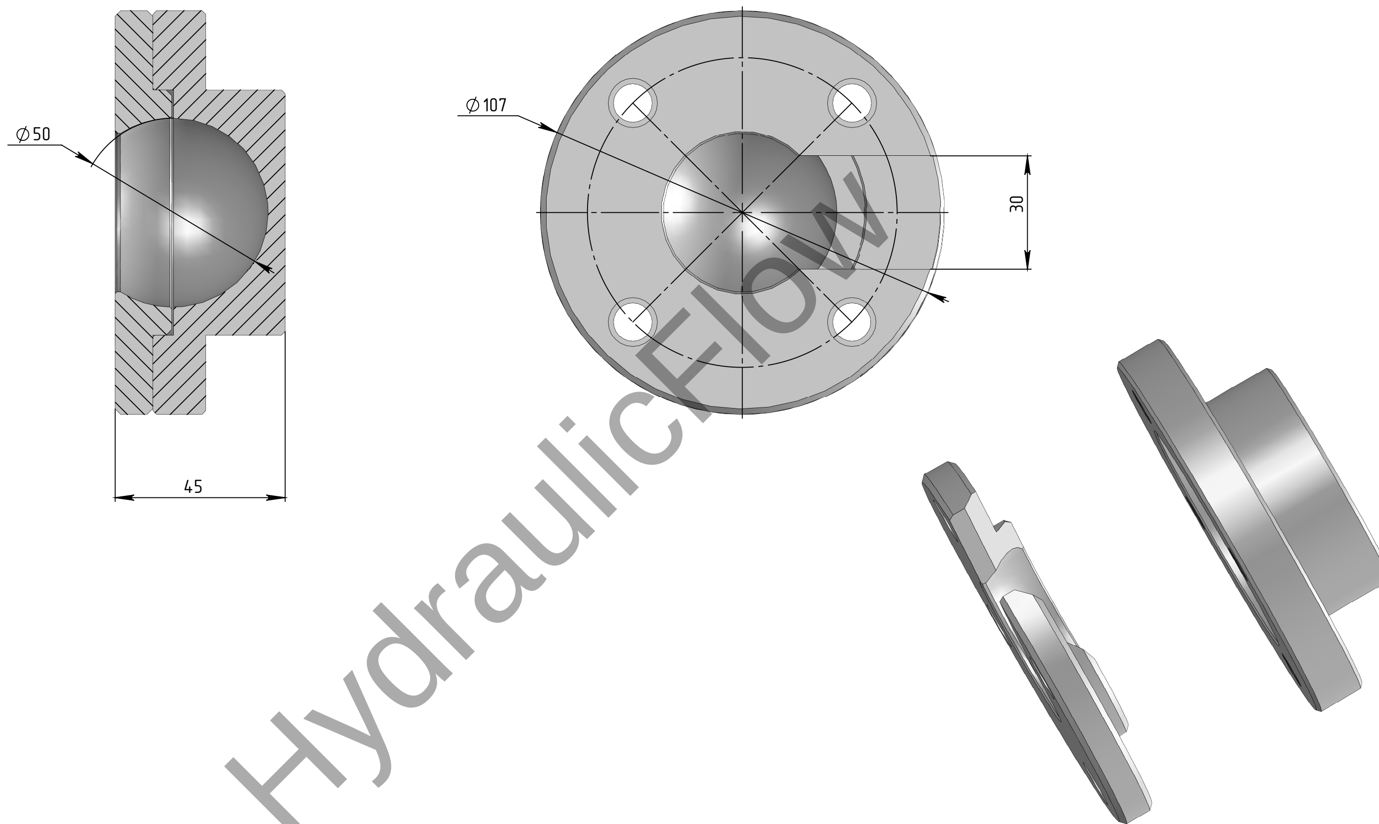
Площадка для встановлення гідроциліндра ГА3-53 СА3
